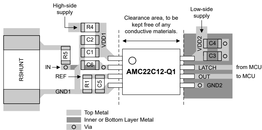
图 10-1. 建议布局 AMC22C12-Q1
