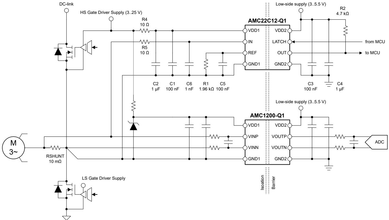
图 8-1. 使用 AMC22C12-Q1 进行过流检测
