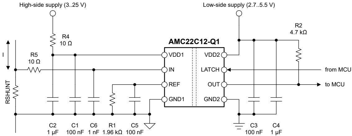
图 9-1. 去耦 AMC22C12-Q1
