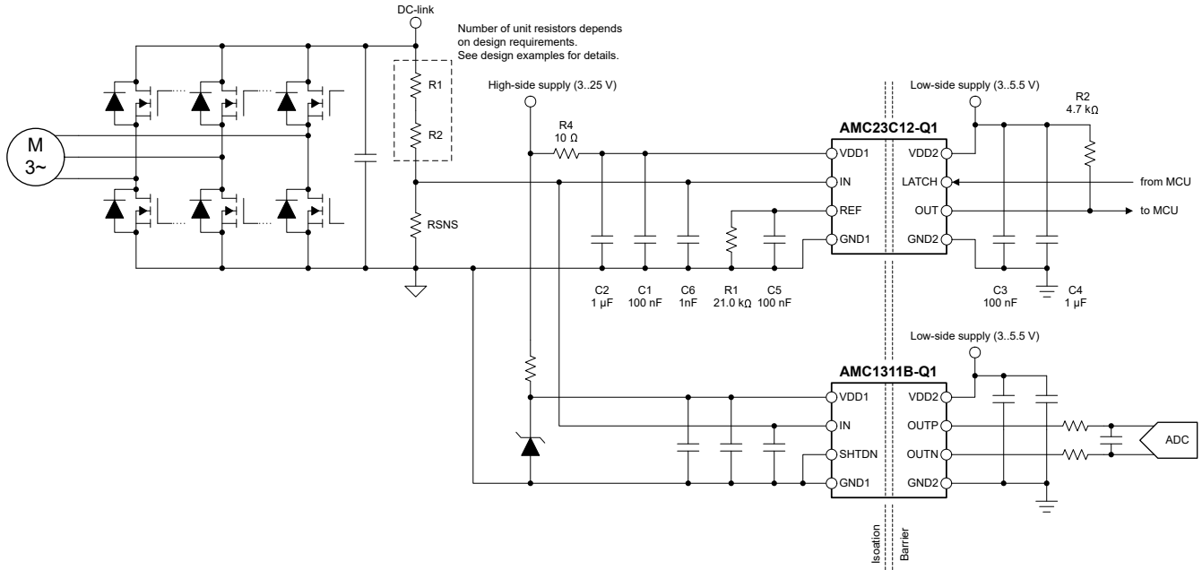
图 8-2. 使用 AMC23C12-Q1 进行过压检测
