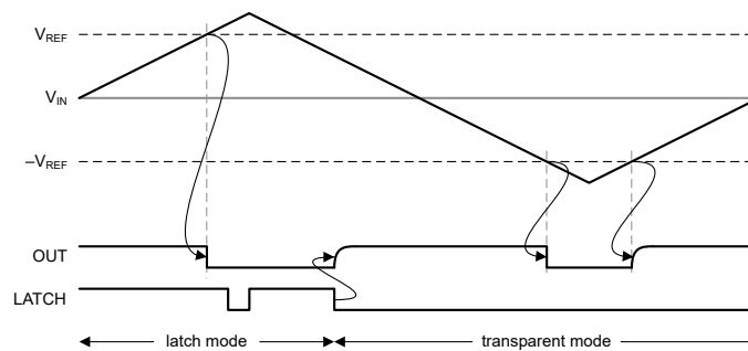
图 6-2. 功能时序图
