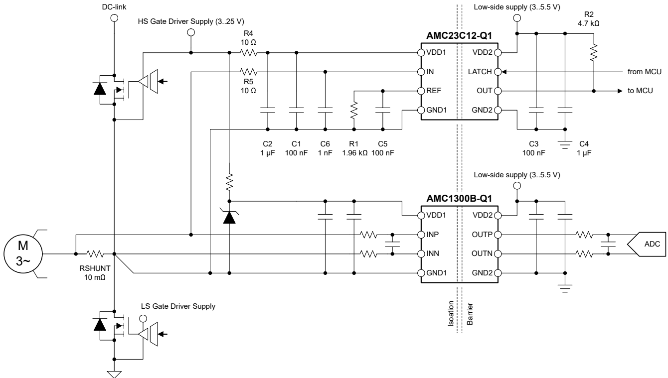
图 8-1. 使用 AMC23C12-Q1 进行过流检测
