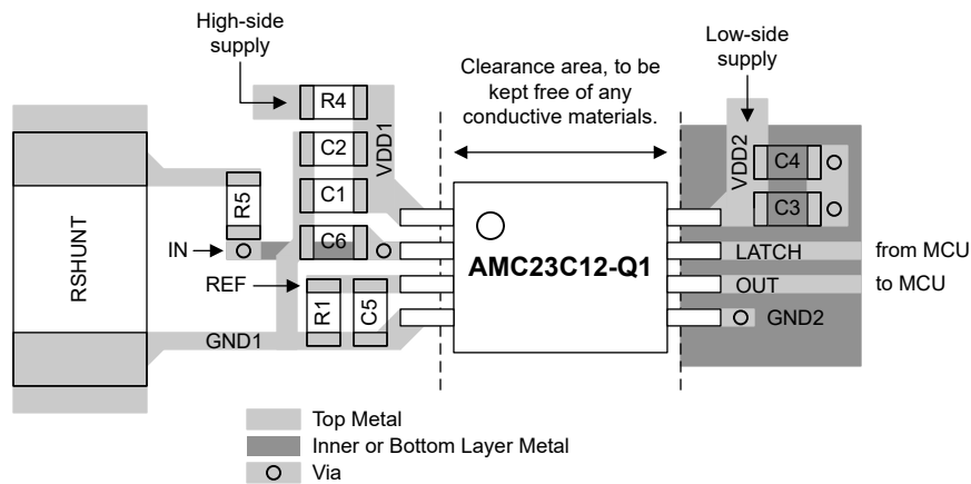
图 10-1. 建议布局 AMC23C12-Q1
