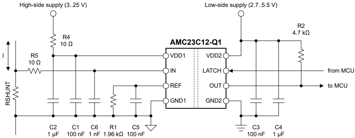
图 9-1. 去耦 AMC23C12-Q1
