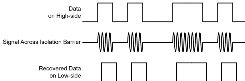
图 7-4. 基于 OOK 的调制方案
