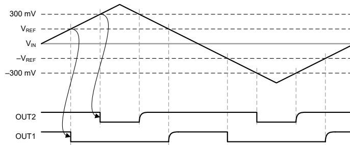
图 6-2. 功能时序图
