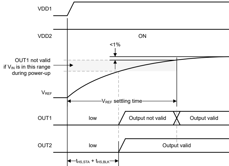
图 7-2. 导致基准电压长建立时间的输出行为
