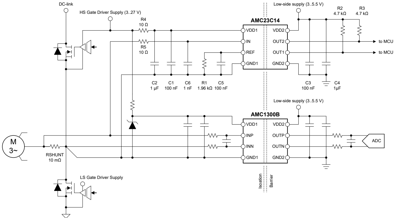
图 8-1. 使用 AMC23C14 进行过流和短路检测
