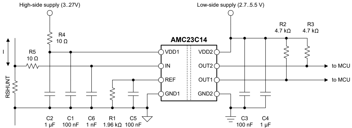
图 9-1. 去耦 AMC23C14
