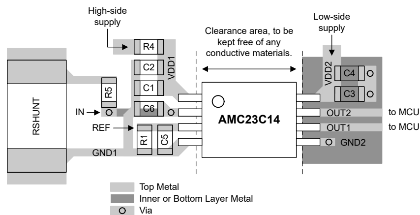
图 10-1. 建议布局 AMC23C14
