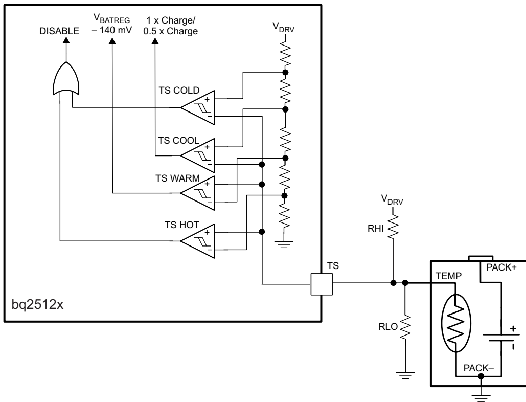
图 18. TS Circuit
