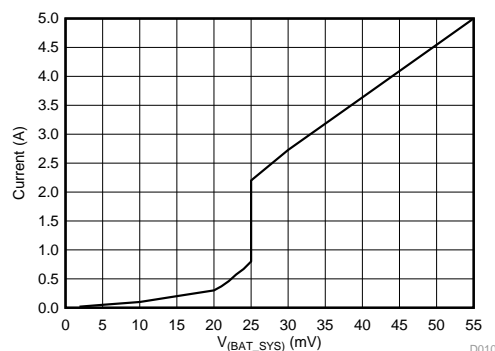
图 12. BATFET V-I Curve
