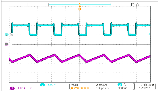
图 56. PWM Switching Waveform
