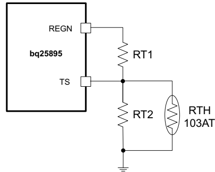
图 14. TS Resistor Network
