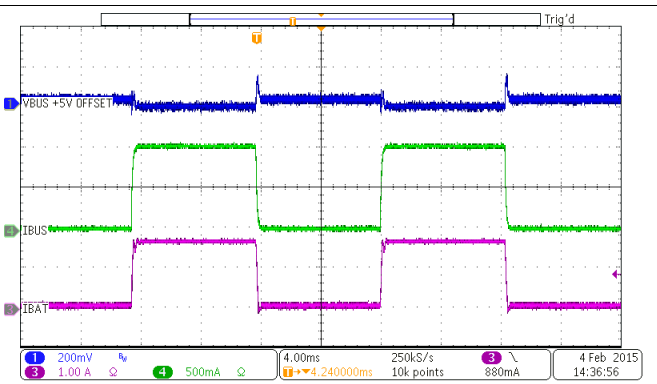
图 57. PFM Switching Waveform
