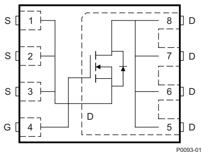
俯视图
