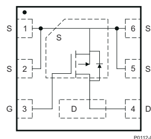
图 3-1. 顶视图
