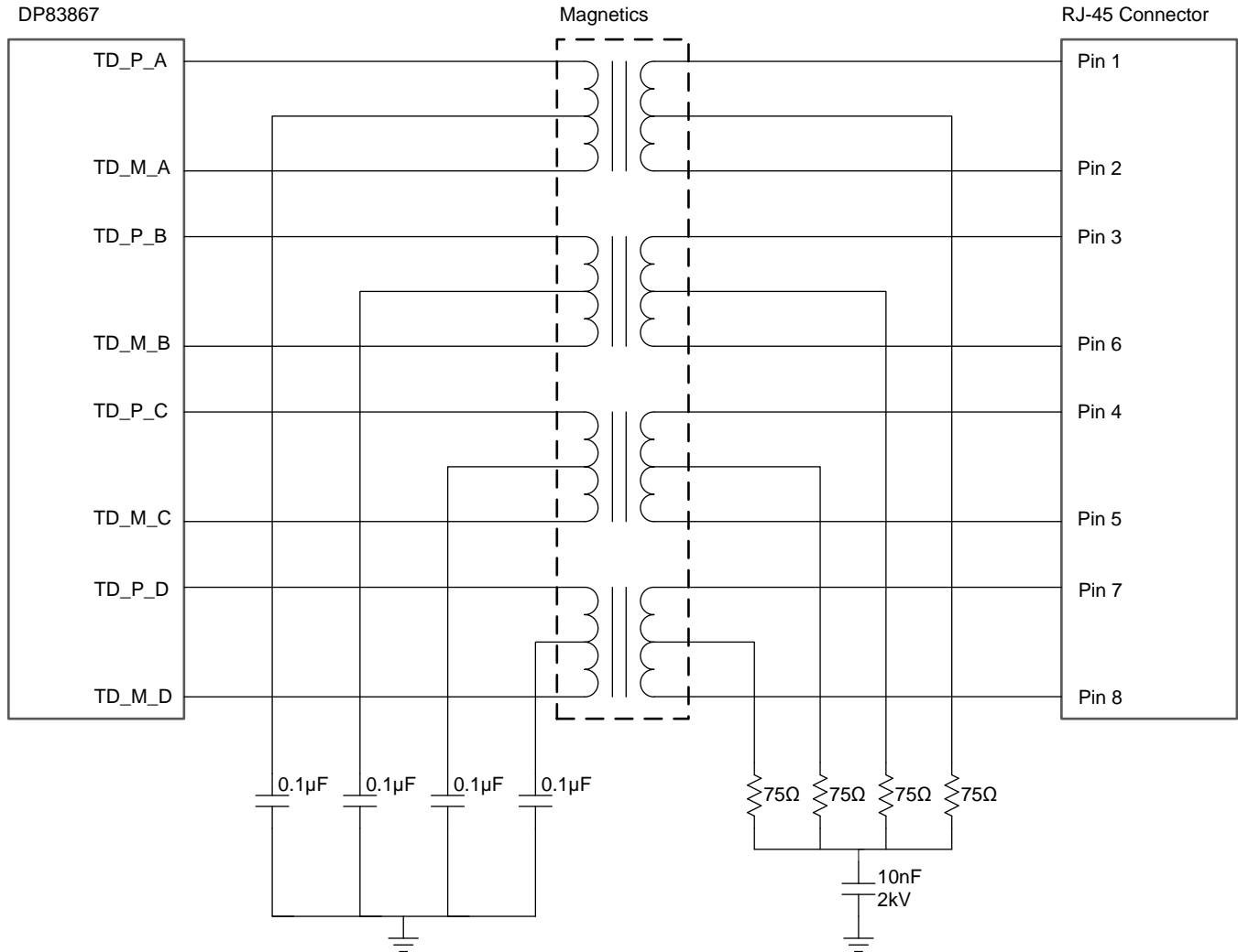
图 26. Magnetics Connections
