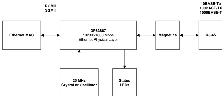
系统图
