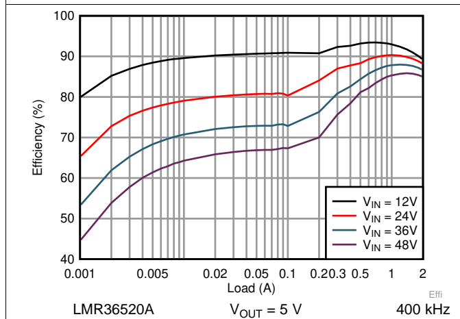
图 18. Efficiency
