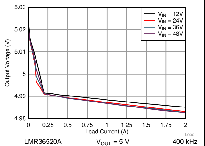
图 19. Load Regulation
