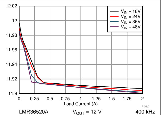
图 21. Load Regulation
