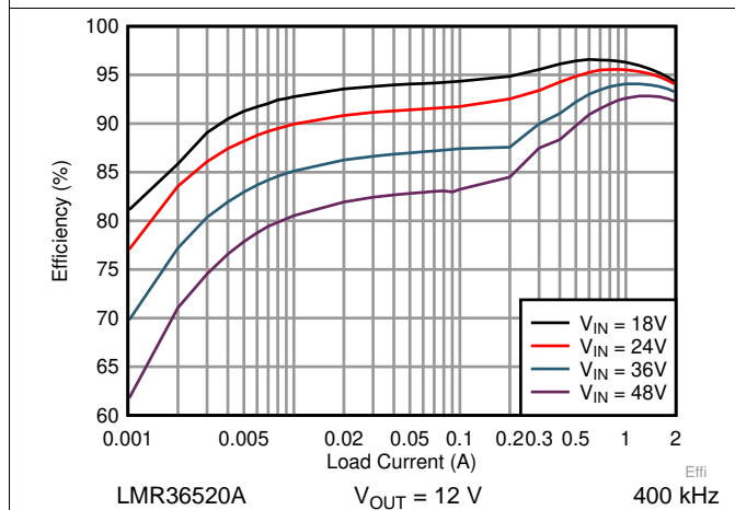
图 20. Efficiency
