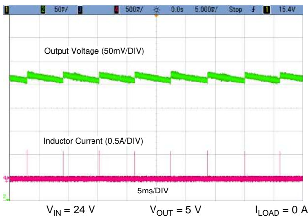
图 30. Output Ripple at No load
