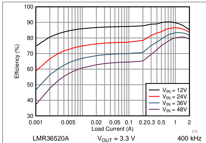
图 16. Efficiency
