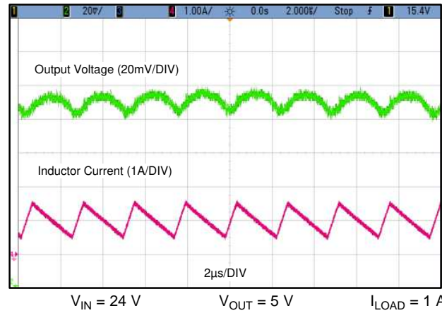
图 31. Output Ripple at 1 A
