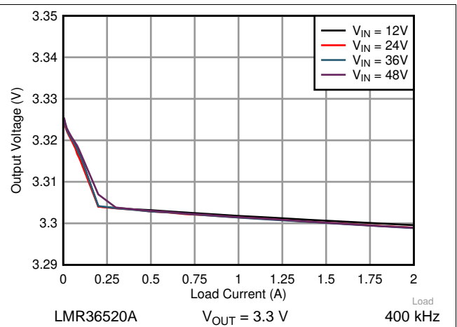
图 17. Load Regulation
