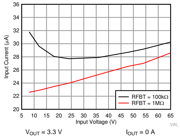
图 24. Input Supply Current
