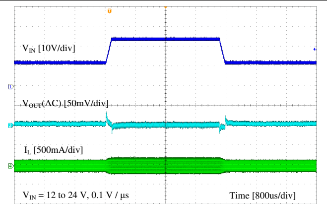
图 9-8. Line Transient
