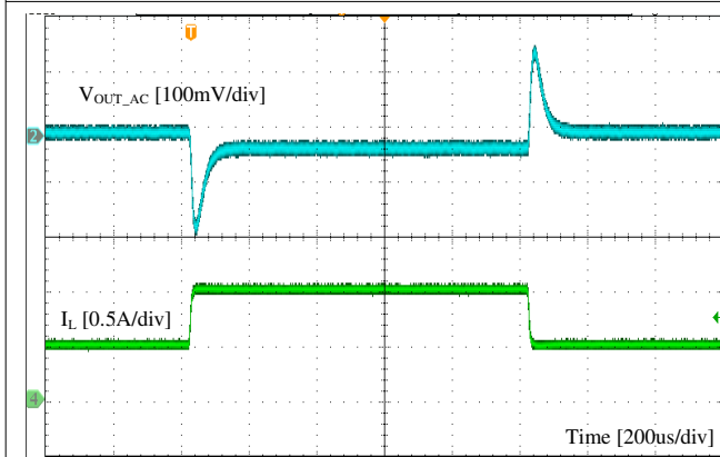
图 9-7. Load Transient
