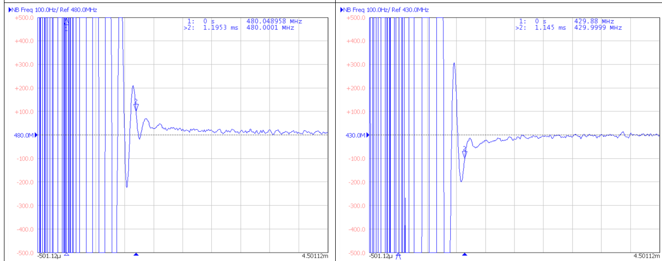
Figure 75. F1 to F2 Switching Time
