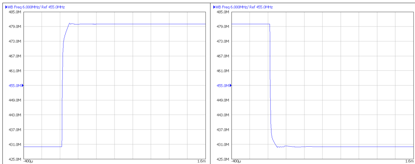
Figure 73. F1 to F2 Switching
