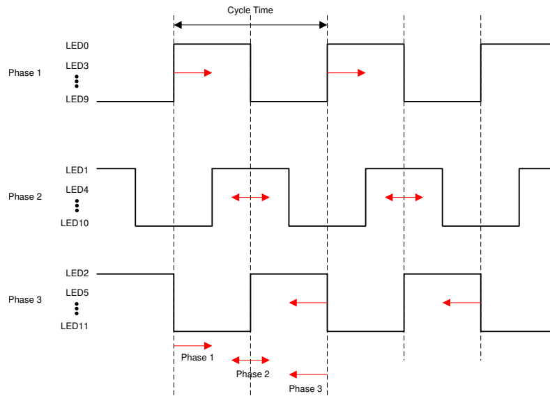
图 12. PWM Phase-Shifting
