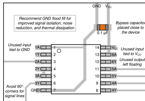
图 11. Example layout for the SN74HCS04-Q1
