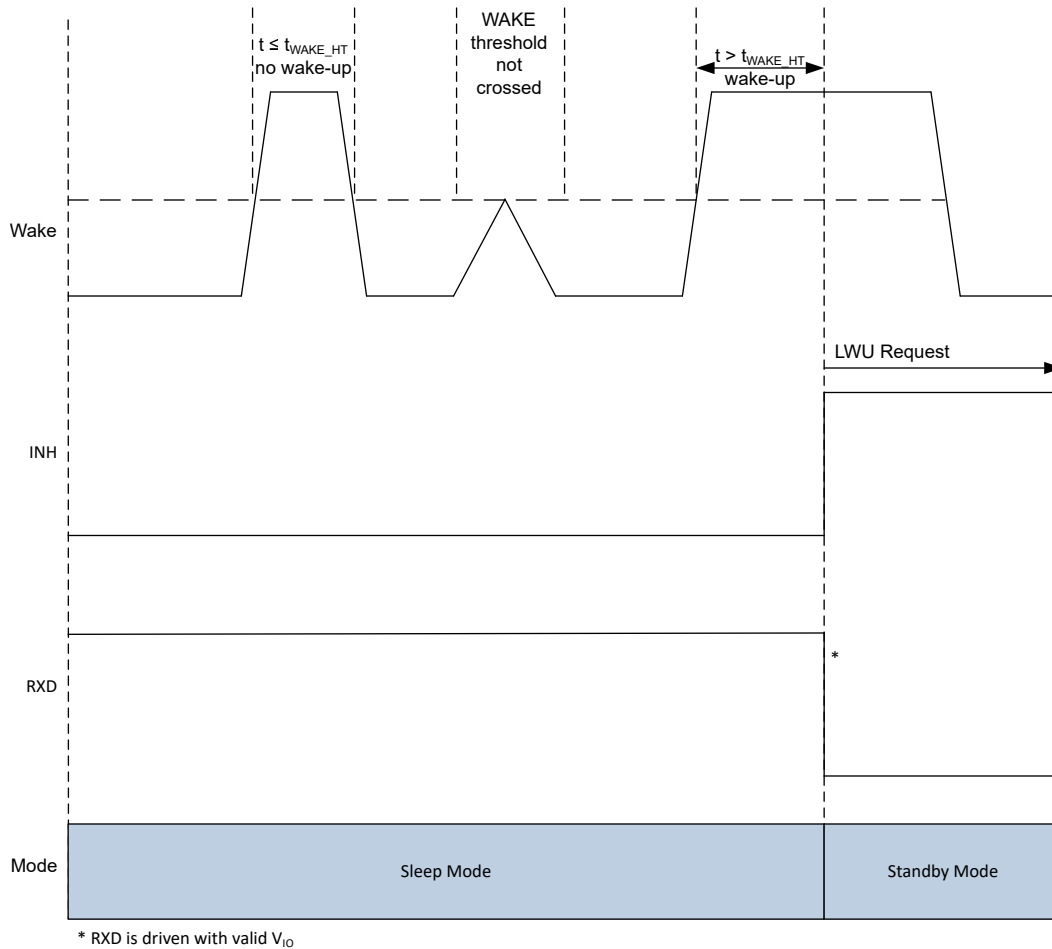
图 8-7. LWU Request Rising Edge
