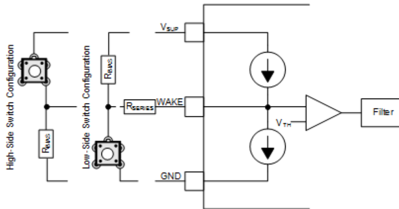
图 8-6. WAKE Circuit Example
