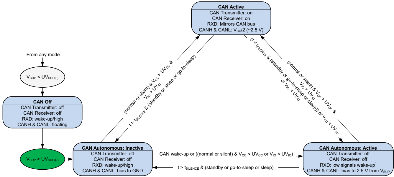
图 8-9. TCAN1043A-Q1 CAN Transceiver State Machine
