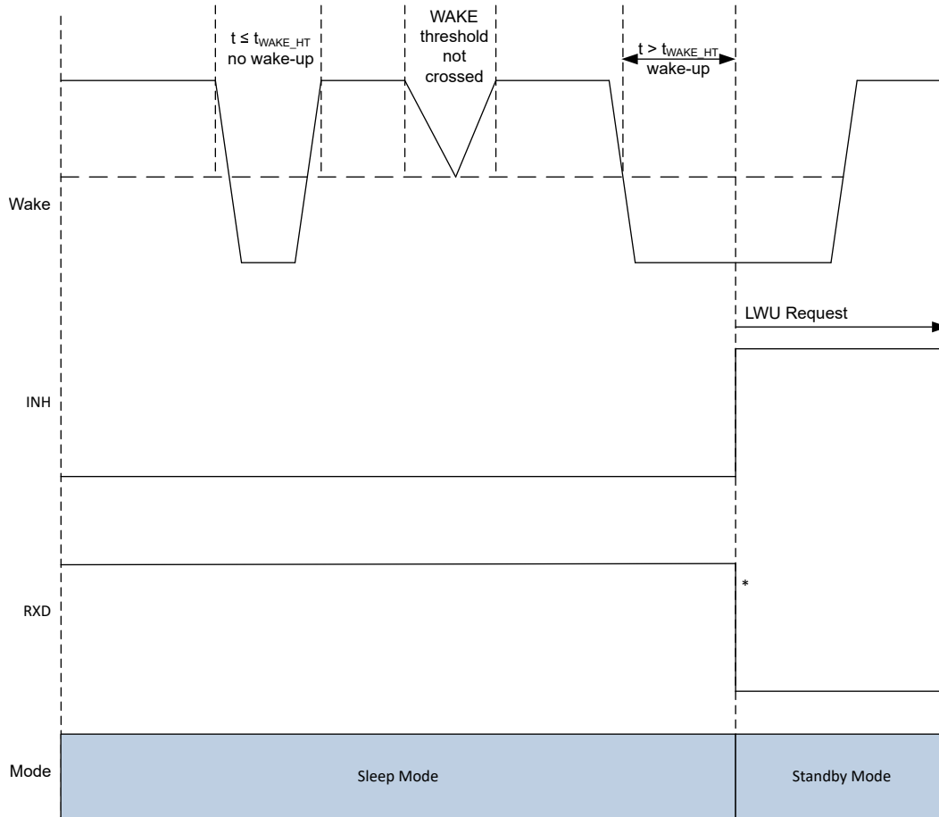
图 8-8. LWU Request Falling Edge
