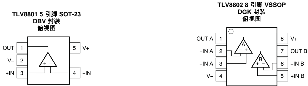
引脚功能：TLV8801 DBV
