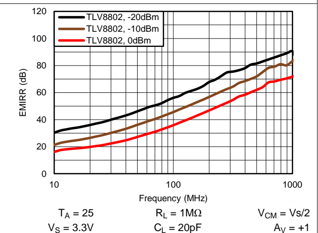
Figure 36. EMIRR 性能
