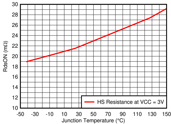
图 6-1. High-Side FET RdsON
