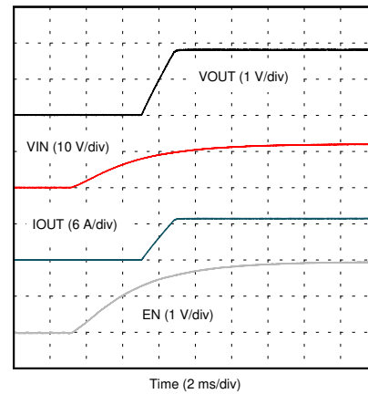
图 8-17. EN Start-Up - DCM
