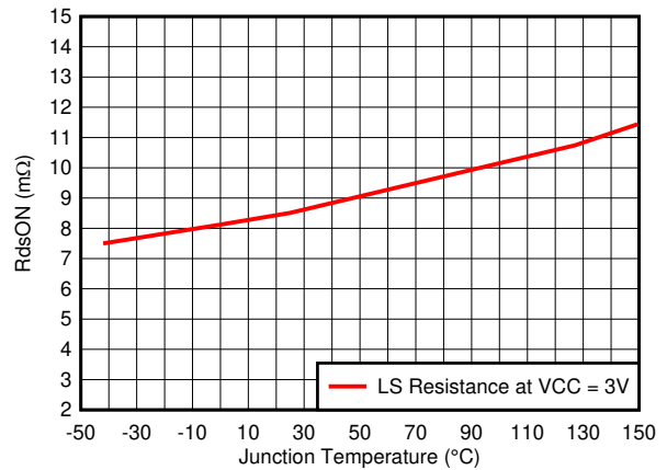
图 6-2. Low-Side FET RdsON
