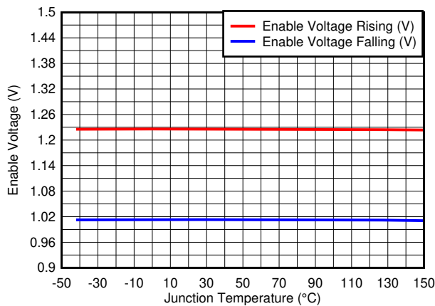
图 6-5. Enable Voltage
