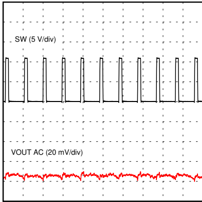
图 8-26. Output Voltage Ripple
