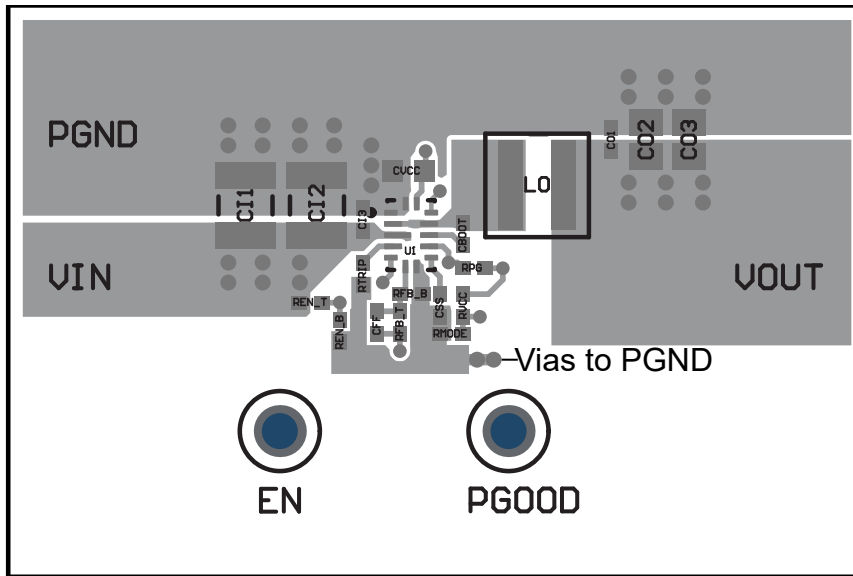
图 10-1. Top Layer Layout
