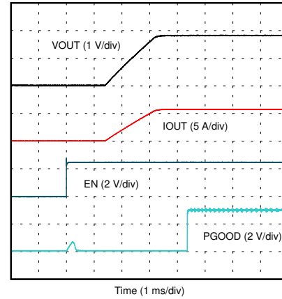
图 8-15. EN Start-Up
