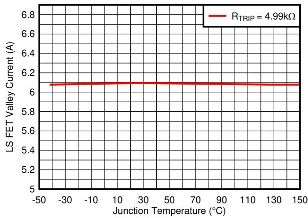
图 6-3. Overcurrent Limit
