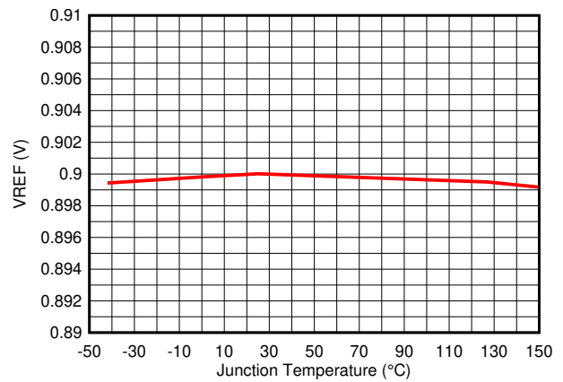
图 6-6. Vref
