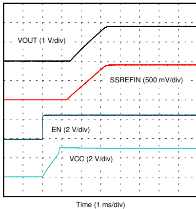
图 8-16. EN Start-Up
