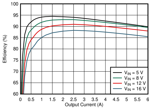
图 8-2. Efficiency - 1100 kHz, FCCM
