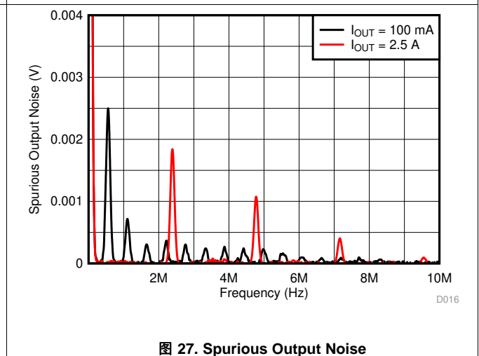
图 27. Spurious Output Noise
